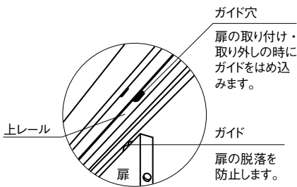
○ (上レール内側) 部分の拡大図
